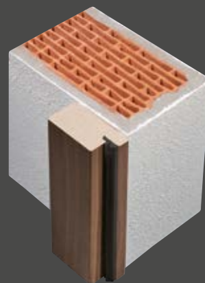
BLENDRAHMEN BM 45 auf der Wand, vor der Laibung montiert
