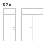
Raumhohe Zarge mit Querteil, Kämpfer und Oberlichte bis Stocklichhöhe von 2.520 mm (einflügelig, zweiflügelig)
