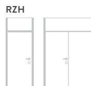
Raumhohe Zarge ohne Querteil mit Kämpfer und Oberlichte bis Raumlichte von 2.600 mm (einflügelig, zweiflügelig)
