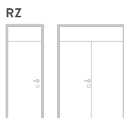
Raumhohe Zarge mit Querteil ohne Kämpfer, mit Oberblende bis Stocklichhöhe von 2.520 mm (einflügelig, zweiflügelig)
