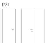
Raumhohe Zarge ohne Querteil und ohne Kämpfer bis Raumlichte von 2.600 mm (einflügelig, zweiflügelig)
